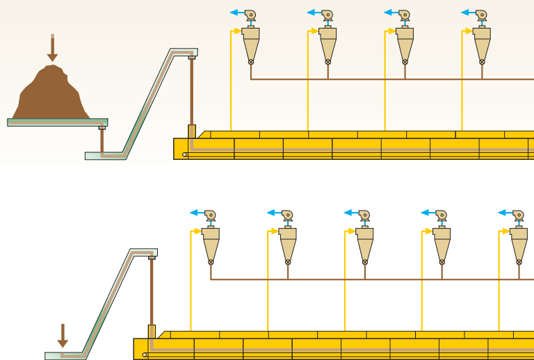
Instalație de uscare
