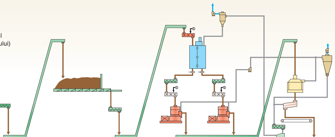
Instalații de peletizat și răcit
