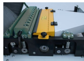
Druckbalken mit Absaughaube
