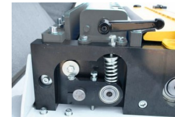
Druckbalken
